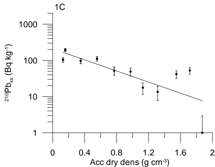
Figur 18. Den bästa kurvanpassningen av ackumulerad torr viktsdensitet och ^{210}\text{Pb} vid station 1.
