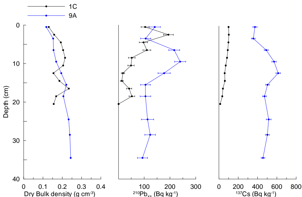
Figur 17. Torrvidktsdensitet, ^{210}\text{Pb} och ^{137}\text{Cs} -aktiviteter i sediment från station 1 och 9. Notera aktivitetsskalan.
