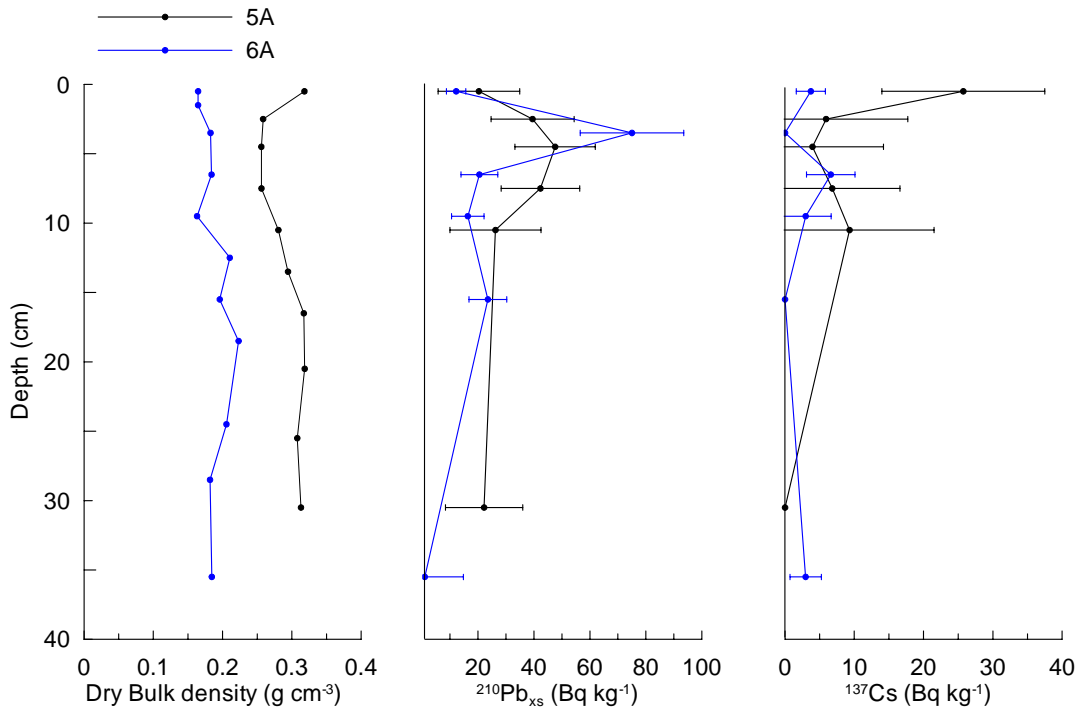
Figur 18. Torr viktsdensitet, ^{210}\text{Pb} och ^{137}\text{Cs} -aktiviteter i sediment från station 5 och 6. Notera aktivitetskalan.
