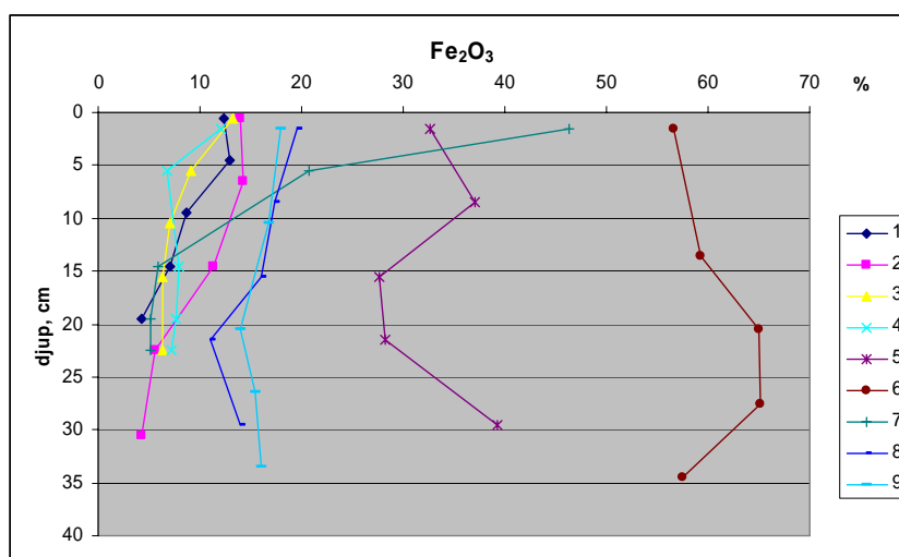
Figur 7. Järninnehållet (vikt % av TS) i sedimenten på olika djup i respektive station uttryckt som \text{Fe}_2\text{O}_3 .
